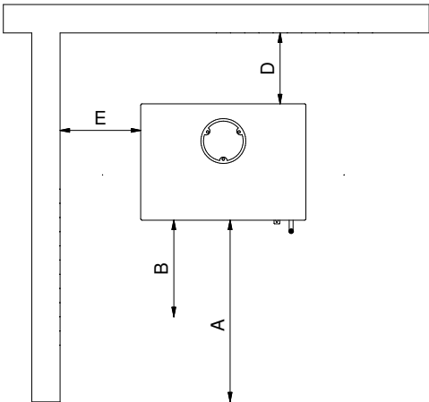
Ohne Strahlungsschutz
