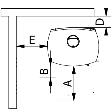
Met reflector
