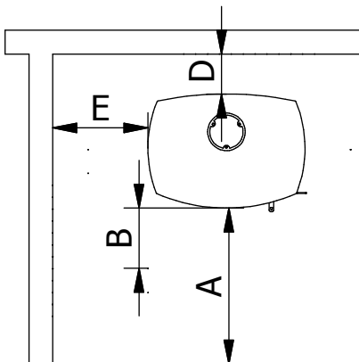
Ohne Strahlungsschutz
