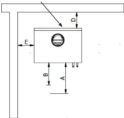
Mit Strahlungsschutz
