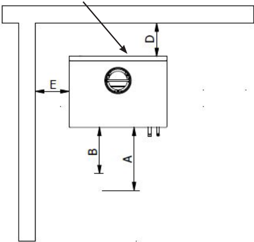
Heijastimella
