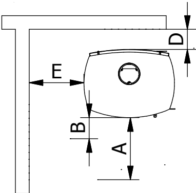
Med reflektor
