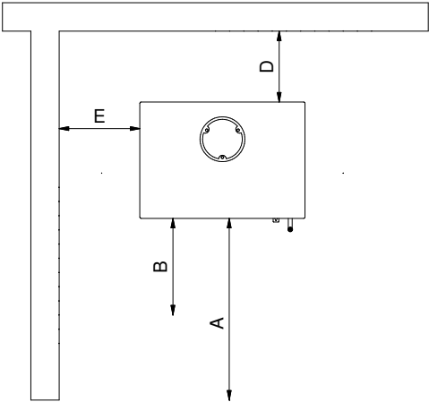
Zonder reflector
