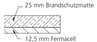
Aufbau von Schrägplatte.
