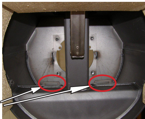
Voorkant van de kachel, van onderaan gezien
