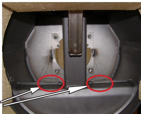
Front af ovn-set nedefra
