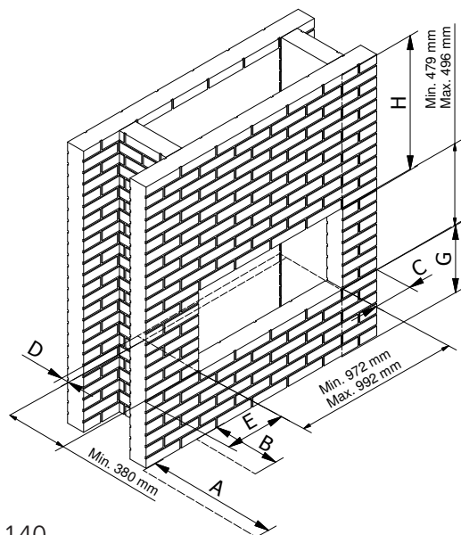
Murs de briques
